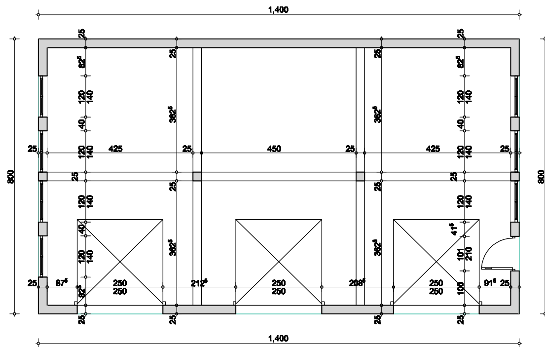
OSNOVA PRIZEMLJA
