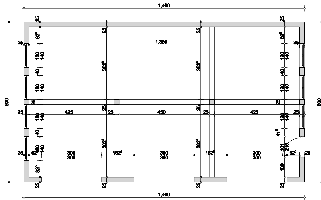
OSNOVA PRIZEMLJA
