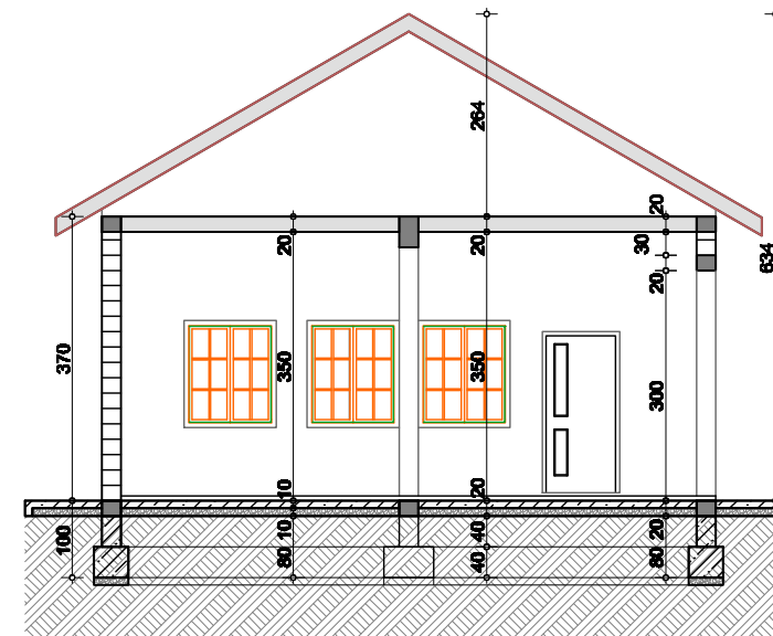
PRESEK
