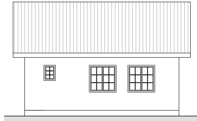
БОЃНИ ИЗГЛЕД 1
