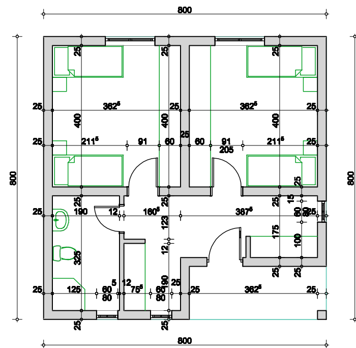
OSNOVA PRIZEMLJA
