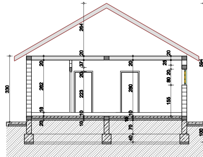
PRESEK
