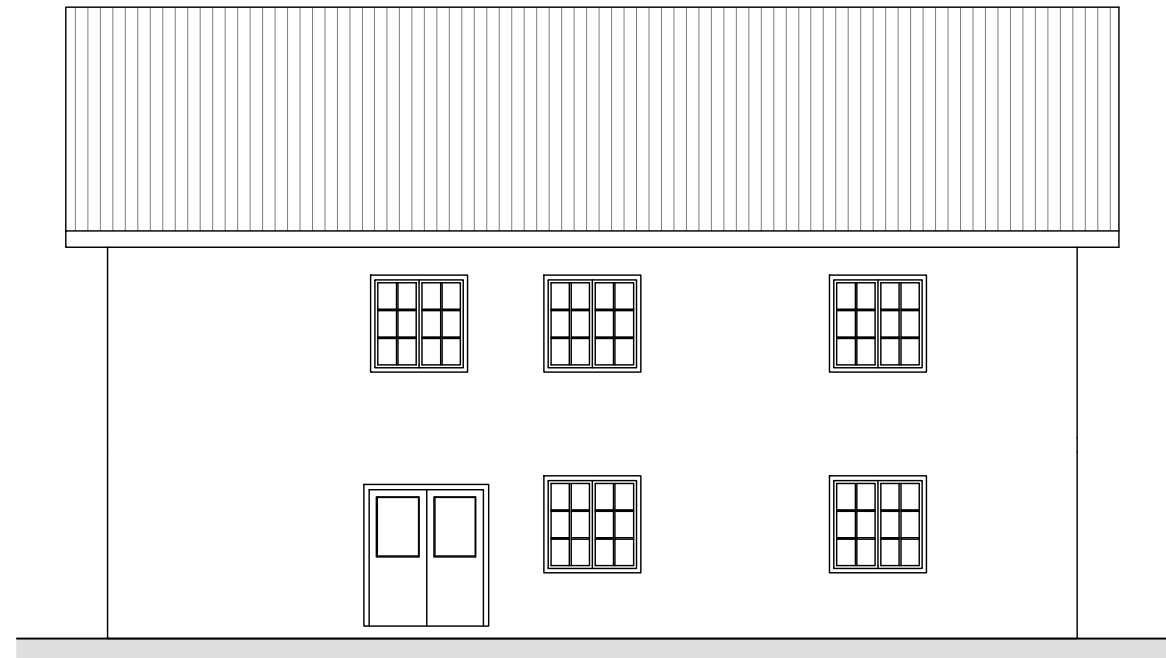
ПРЕДНИ ИЗГЛЕД
